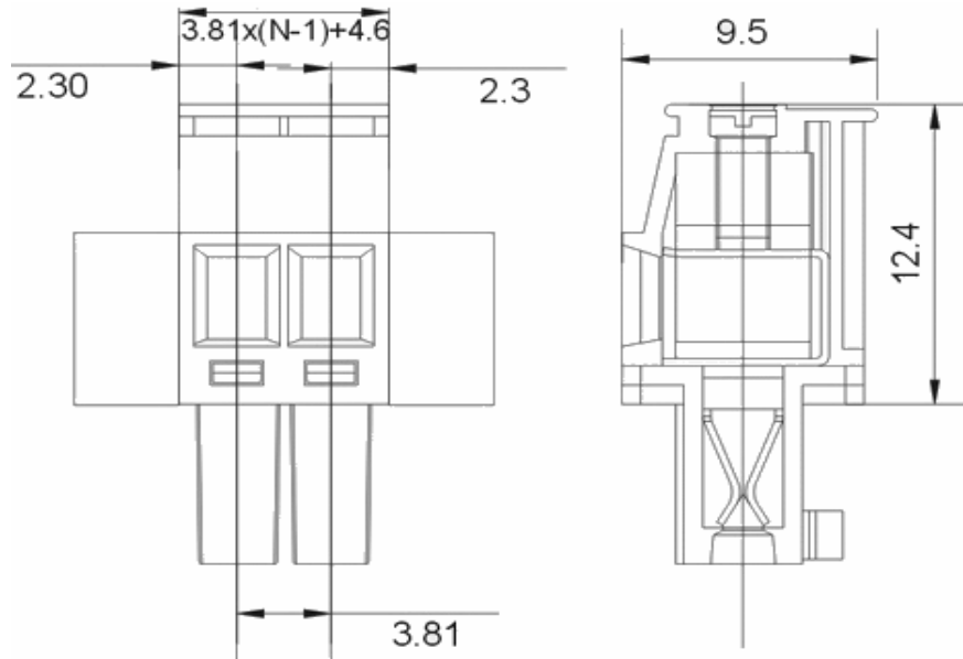
P.C.B. Layout
