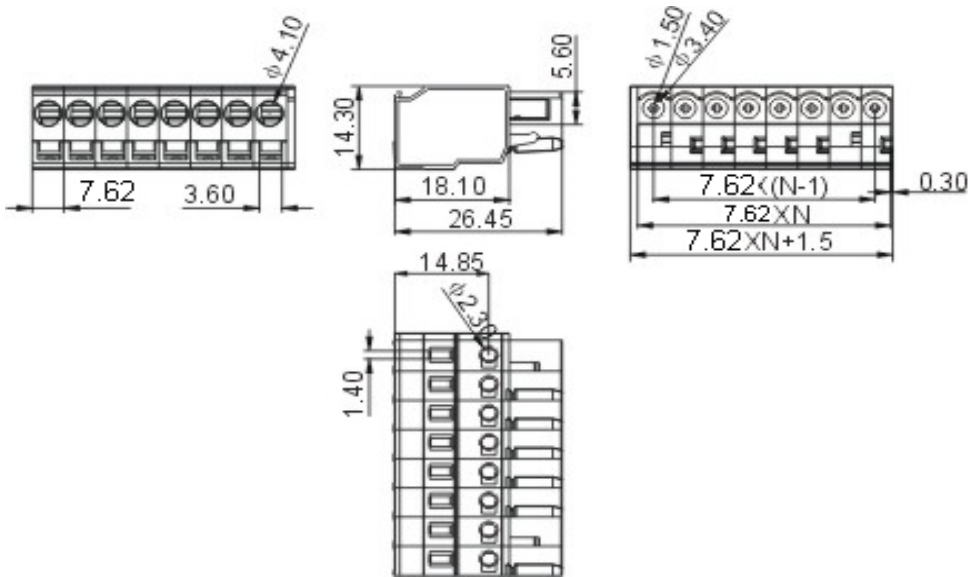
P.C.B. Layout
