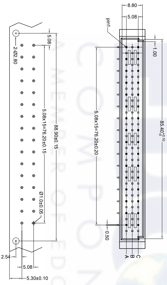
P.C.Board Layout
